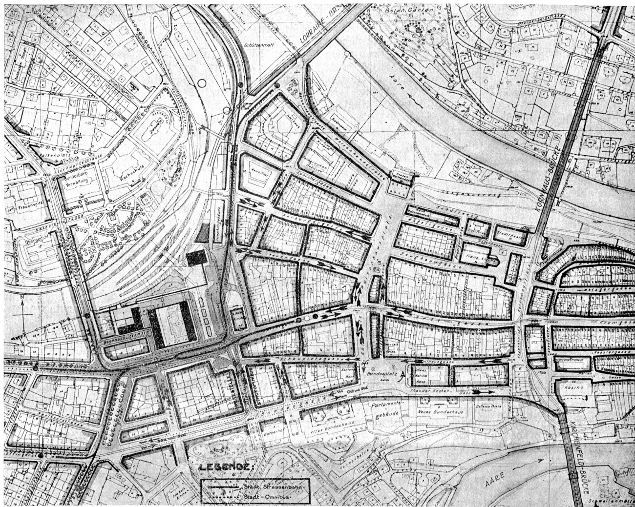
Zum Wettbewerb zu einem Bebauungsplan des Bahnhof- und Bubenbergrasses in Bern. Der im zweiten Rang mit 5000 Fr. preisgekürnte Entwurf von Ingenieur E. Hüttel und Architekt E. Schinler, Zürich (Uebersichtsplan).
