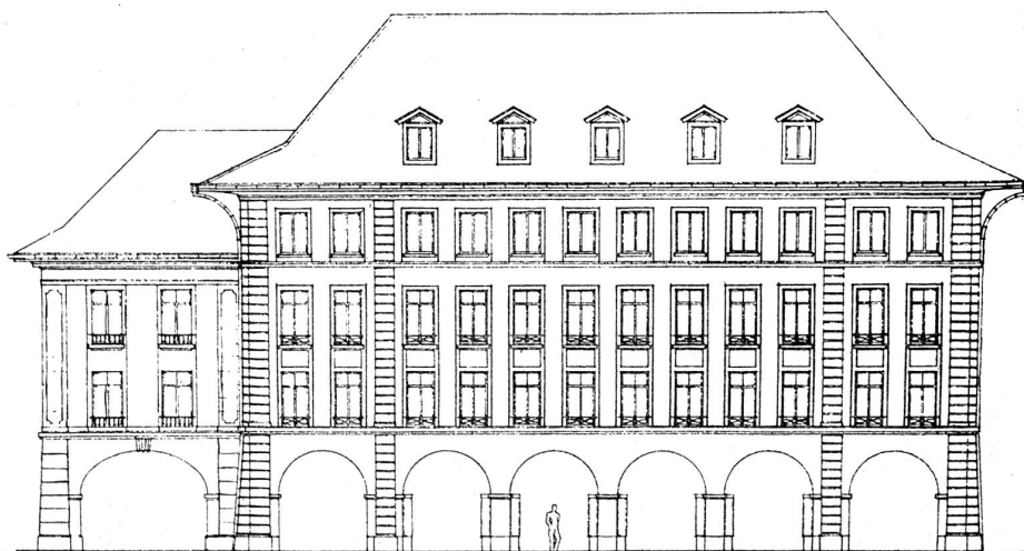
Der erstprämierte Entwurf der Architekten Zeerleder und Wildbolz. Blick gegen den neu zu erstellenden Anbau südlich des Hôtel de Musique.
