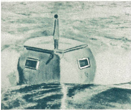
In Einer-Unterseeboot hat der amerik. Ingenieur Farney Connat aus Chicago erfolgreich konstruiert. Es hat eine Länge von wenig über drei Meter. Die Besatzung besteht nur aus dem Konstrukteur Connat. Das Boot ist hier tauchbereit. (Phot. Keystone)
