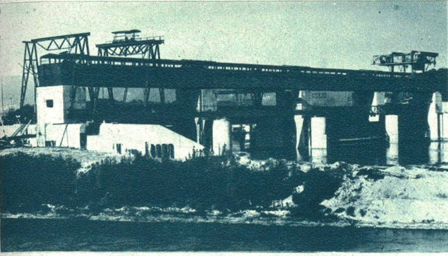
Die Bauarbeiten für das Aarekraftwerk Döttingen-Klingnau schreiten rasch vorwärts. Die Ausmaße dieses im Entstehen begriffenen Großkraftwerkes übertreffen die üblichen Dimensionen. Unser Bild links zeigt das im Bau begriffene Turbinenwerk des Kraftwerkes Döttingen-Klingnau. — Unser Bild rechts zeigt eine Gesamtansicht des neuen Kraftwerkes Albbruck-Dogern oberhalb Laufenburg, welches in Betrieb genommen wurde. Die Rheinstaung beträgt volle zwei Meter. Photopress, Zürich.
