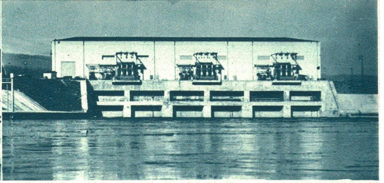
Die Bauarbeiten für das Aarekraftwerk Döttingen-Klingnau schreiten rasch vorwärts. Die Ausmaße dieses im Entstehen begriffenen Großkraftwerkes übertreffen die üblichen Dimensionen. Unser Bild links zeigt das im Bau begriffene Turbinenwerk des Kraftwerkes Döttingen-Klingnau. — Unser Bild rechts zeigt eine Gesamtansicht des neuen Kraftwerkes Albbruck-Dogern oberhalb Laufenburg, welches in Betrieb genommen wurde. Die Rheinstaung beträgt volle zwei Meter. Photopress, Zürich.
