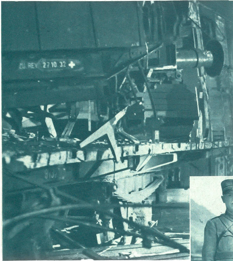
Der auf den nachfolgenden Drittklasswagen gestoßene Gepäckwagen des Eilzuges Zürich—Uster. Photo K. Egli, Zürich.
