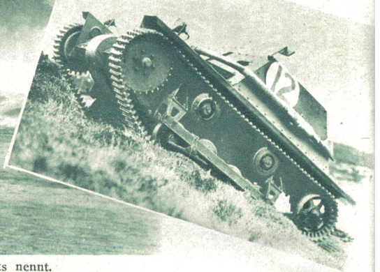
Oben rechts: Der »Windhund-Tank«, eine neue Waffe der englischen Armee. Die Tanks bewältigen Steigungen von 1 zu 3 spielend und zeigen selbst beim Erklettern von Dämmen und Hügeln ungewöhnliche Schnelligkeiten.
