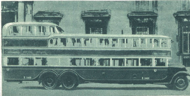
Ein Autobus-Ungetüm. Ein dreistöckiger Autobus, den die Stadt Rom für den Ausflugsverkehr nach Tivoli bauen ließ. Das Monstrum ist 12 m lang, 3,5 m hoch und kann 88 Passagiere fassen. Der Wagen ist hergestellt aus dem für den Fahrzeugbau immer mehr verwendeten leichten Duraluminium.
