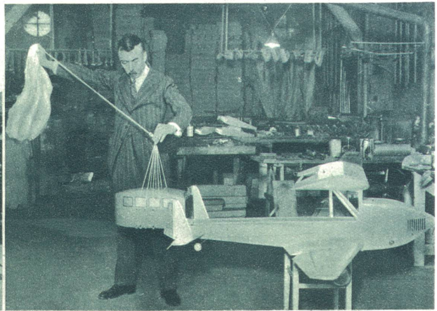
Ein neuartiges Flugzeugmodell, das unter Aufsicht des französischen Luftfahrtministeriums ausprobiert wird. Die Kabine ist beweglich, kann auf dem Gestell nach rückwärts verschoben werden, um bei Unfällen die Passagiere leichter mit Fallschirmen retten zu können.
