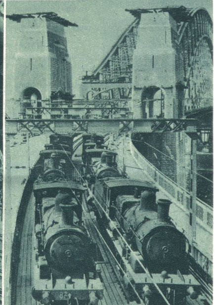
Brückenprobe. Die Tragfähigkeit der kürzlich eröffneten Riesenbrücke über den Golf von Sydney (Australien) wird durch Belastung mit Lokomotiven (total 400 Tonnen Gewicht) geprüft.
