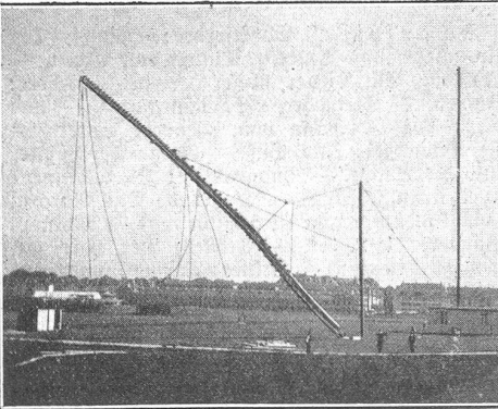
Das obenstehende Bild hält den zweiten Mast während dem Aufziehen fest. Im Hintergrund erkennt man die schlanke Form des ersten, bereits aufgestellten Mastes, dessen definitive Verankerung
