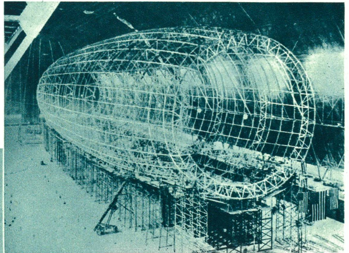
Das Gerippe des künftigen amerikanischen Luftriesen „7 R S — 4“, der gegenwärtig in der Bauhalle von Akron (Ohio) montiert wird. Mit einer Länge von über 260 Meter wird „7 R S — 4“ das größte Luftschiff der Welt sein.
