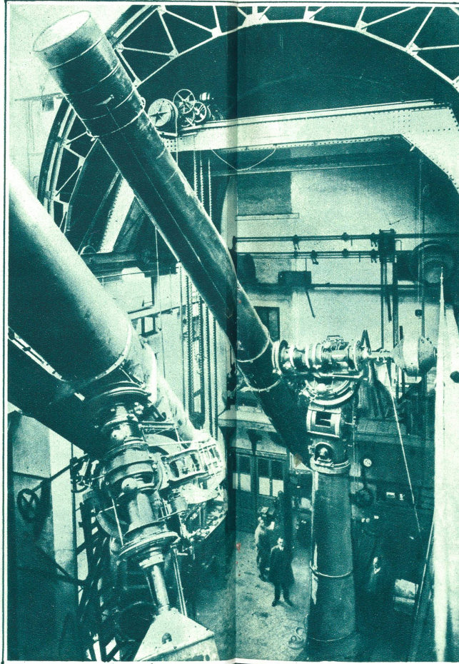
Ein Riesenfernrohr auf dem Montagestand der berühmten Zeiß-Werke in Jena, bestimmt für die Sternwarte in Belgrad.
