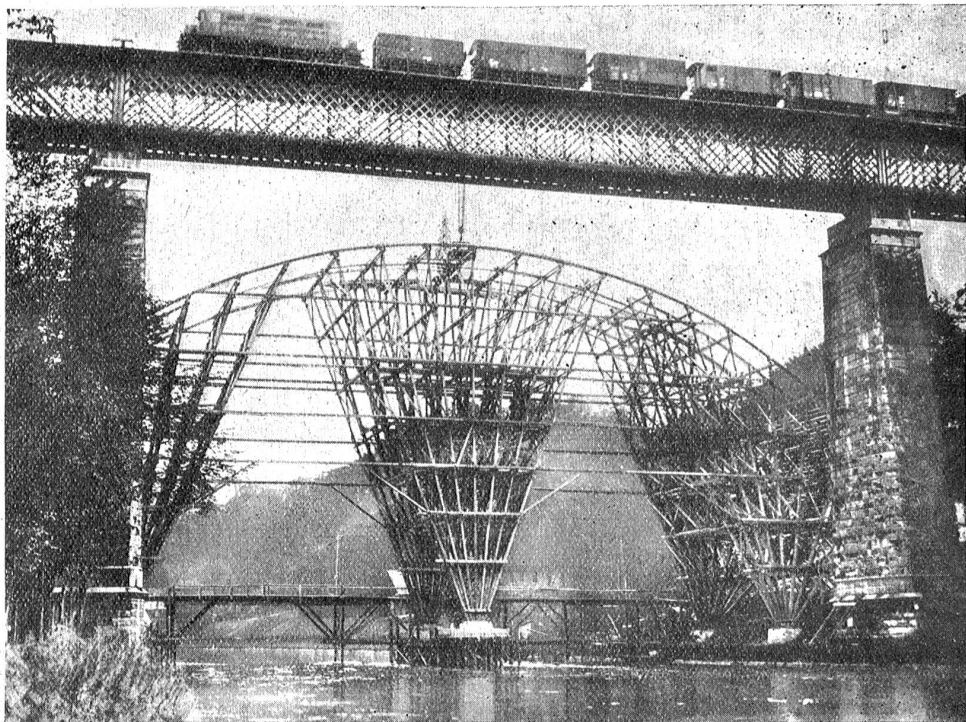
Von der Lorrainebrücke. — Gegenwärtiges Baustadium.
