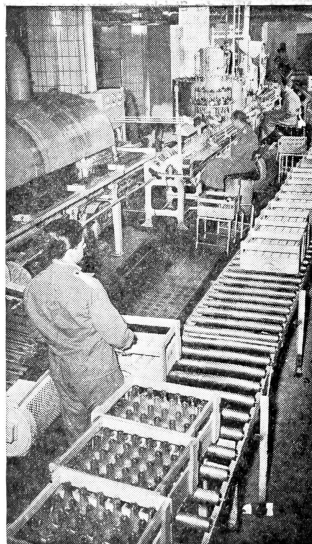
Teilansicht des Maschinensals von der Waschmaschine bis zur Korkmaschine.
