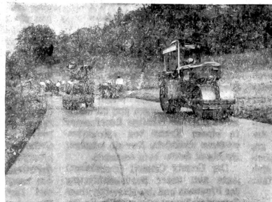
Straße Regensdorf-Wettingen Asphaltteerbetonbelag 3 cm
