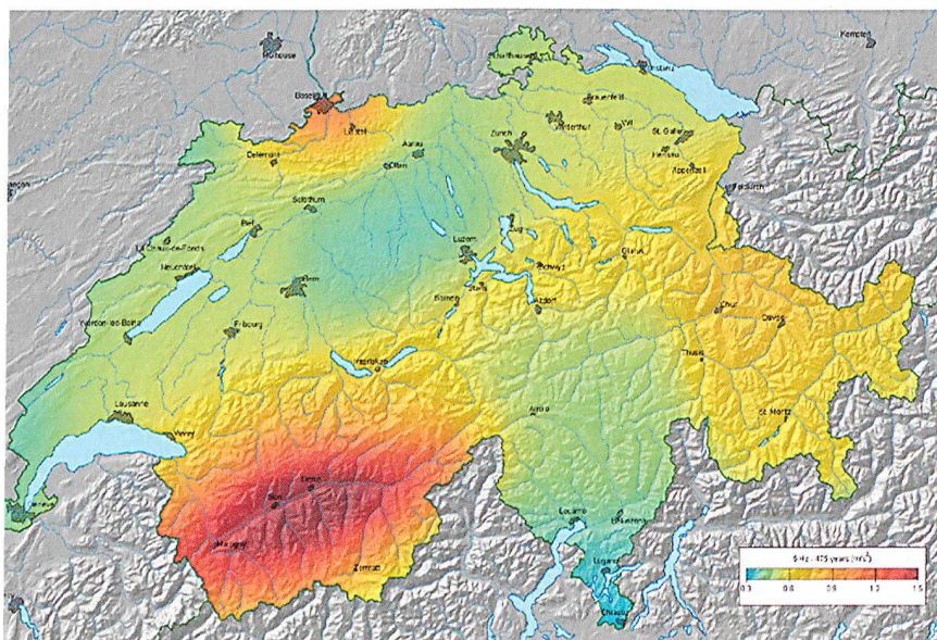
Erdbebengefährdung der Schweiz: Das Wallis, die Region Basel, die Zentralschweiz, das St. Galler Rheintal und das Engadin weisen eine erhöhte Erdbebenaktivität und damit eine signifikante Gefährdung auf.
