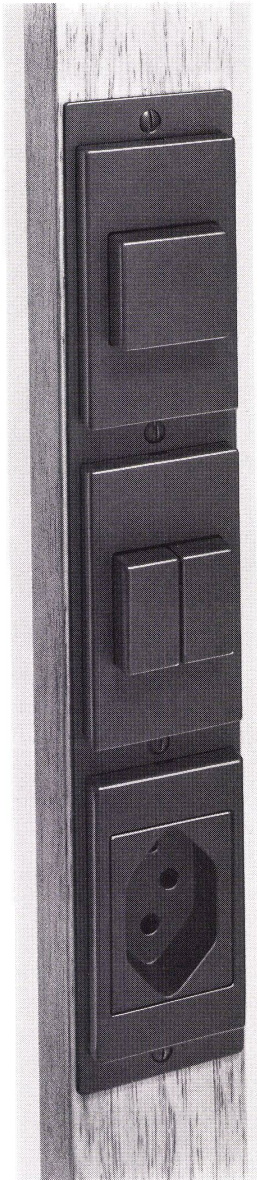
FLF-Apparate in Türzarge eingebaut
