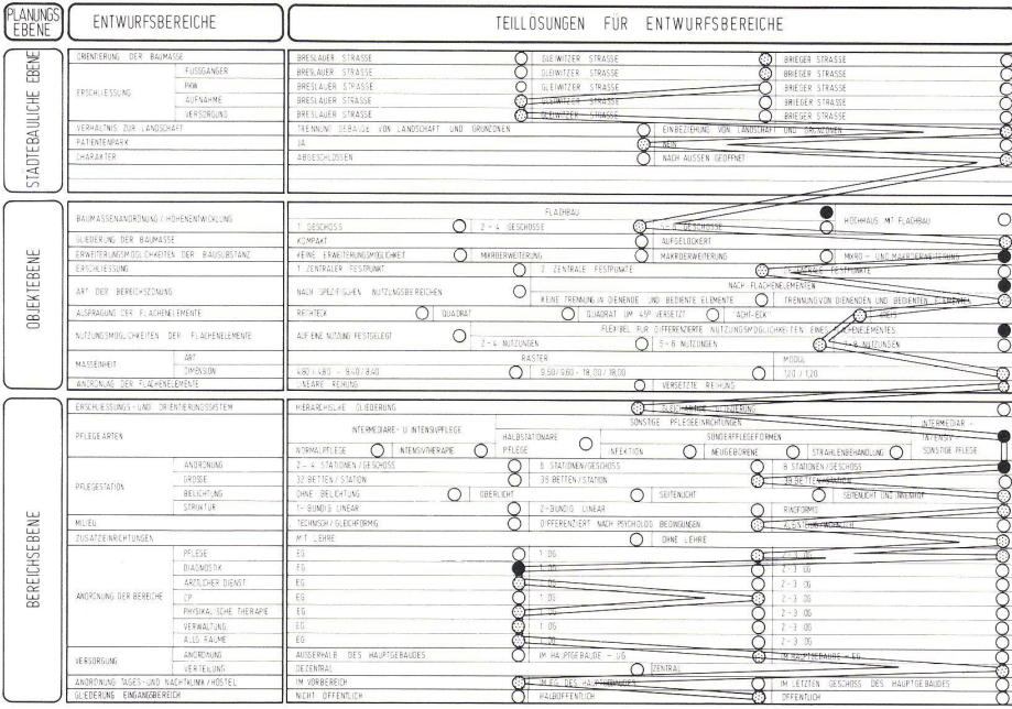
6 Morphologischer Kasten, gegliedert in Entwurfsebenen, mit Lauffinie des Lösungstyps. Éléments morphologiques organisés au niveau du projet avec ligne de développement de la solution type. Morphological box, articulated into design levels, with line of development of typical solution.
