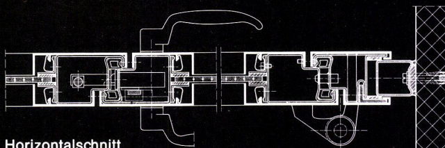
Horizontalschnitt
