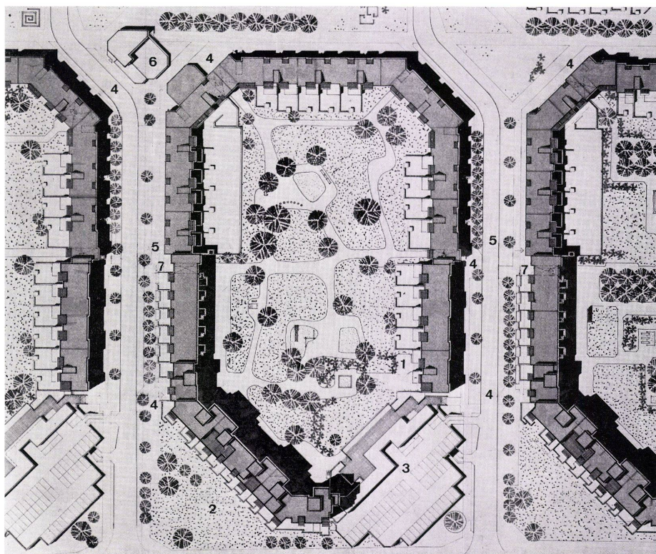
2 Innenhof als Fußgängerbereich mit Kinderspielplätzen. Cour intérieure réservée aux piétons avec aires de jeu pour enfants. Interior courtyard as pedestrian area with children's playgrounds.
