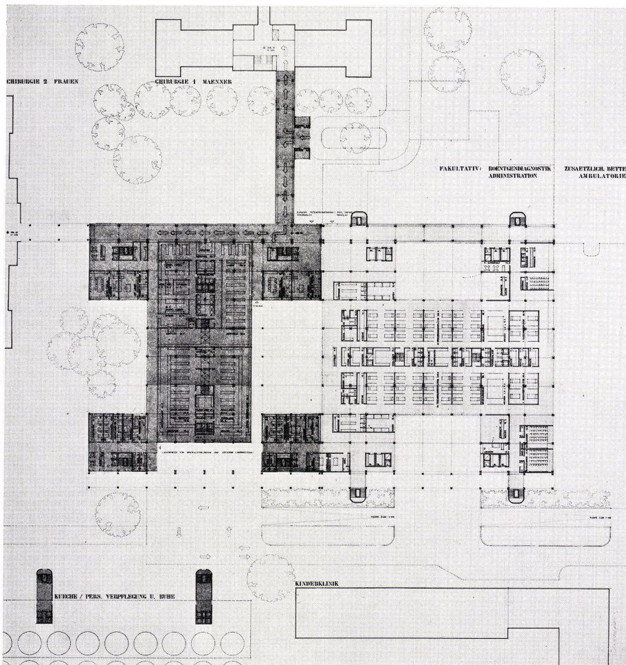
7 Grundriß Erdgeschoß. Eingangsbereich, physikalische Therapie, Zentralsterilisation, Zentralapotheke. Plan du rez-de-chaussée. Zone d'entrée, physico- thérapie, stérilisation centrale, pharmacie centrale. Plan of ground-floor. Entrance zone, physiotherapy, central sterilization, central pharmacy.
