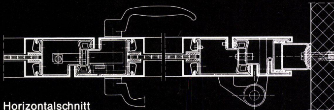
Horizontalschnitt
