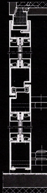
Vertikalschnitt
