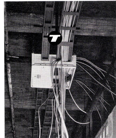
Zwischendecken-Installation
