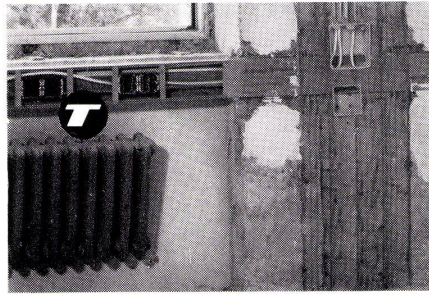
Einspeisung Starkstrom + Schwachstrom
