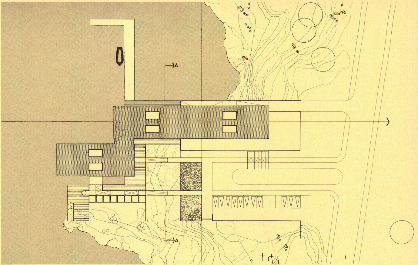
3 Geschosßplan des Hotelprojektes 1:1000. Plan d'étage de l'hôtel projeté. Floor plan of the hotel.
