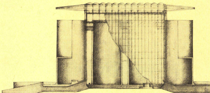
3 Schnitt. Coupe. Section.
