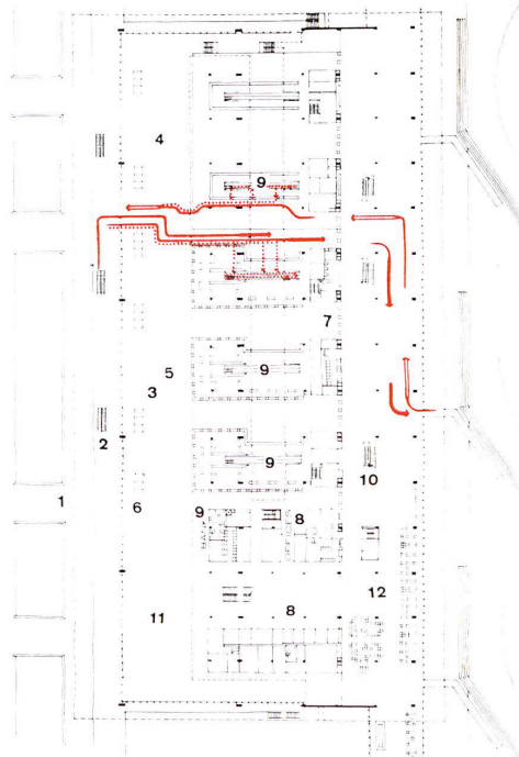
3 Grundriß des Hauptgeschosses 1:2000. Plan de l'étage principal. Plan of main level.
