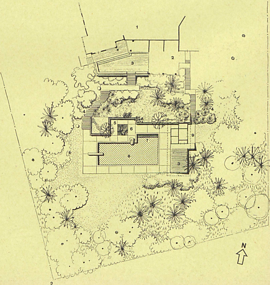
2 Grundriß 1:400. Plan. 1 Haus / Maison / House 2 Garage 3 Holzterrasse / Terrasse en bois / Wooden terrace 4 Stufen / Marches / Steps 5 Skulpturierte Wand / Paroi sculptée / Sculptured wall 6 Steinmosaik / Mosaïque en pierres / Stone mosaic 7 Wasserspeier / Jet d'eau / Fountain 8 Schwimmbecken mit Sprungbrett / Piscine avec tremplin / Swimming-pool with diving-board 9 Toiletten und Filteranlage / Toilettes avec filtre / Toilets and filter plant
