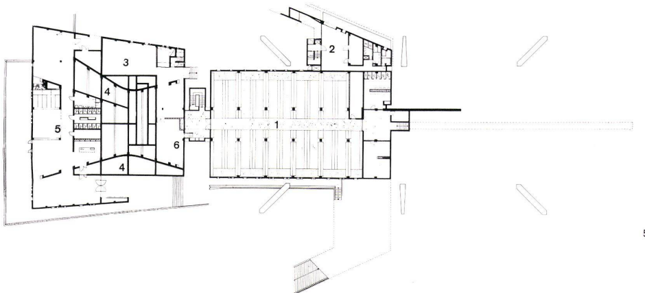
5 Seite / page 261 Westecke des Golfhauses mit Treppenturm. Angle ouest du club. West corner of clubhouse.
