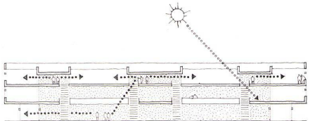
Längsschnitt / Coupe verticale / Longitudinal section
