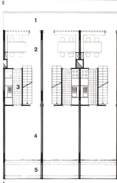
2 Grundriß 1:150 der 2-Raum-Wohnungen im 1. und 6. Obergeschoss. Der Schlafraum ist als Alkove im Inneren des Hauses angeordnet.
