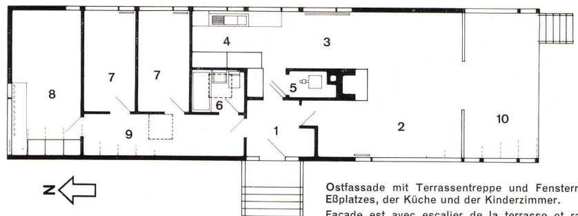
Erdeschoß Grundriß 1:150.
