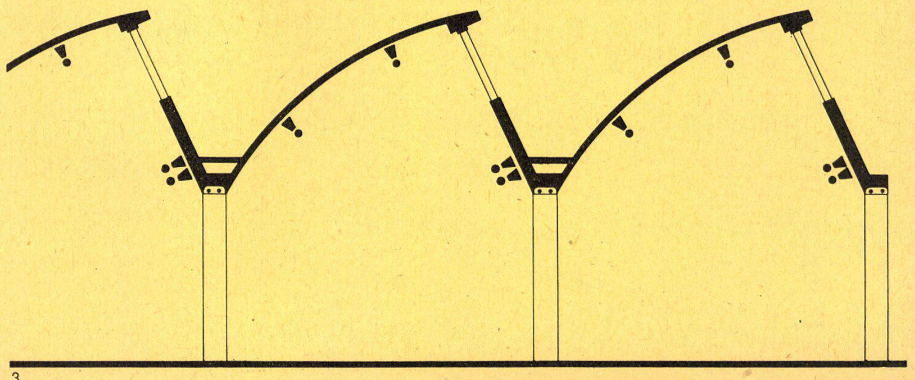
3 Beleuchtungsanordnung in einer Schalenshedhalle. Disposition de l'éclairage de la salle à coquilles shed. Arrangement of illumination in a shell shed hall.
