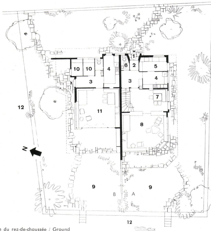
Grundriß Erdgeschoß / Plan du rez-de-chaussée / Ground floor plan 1:250
