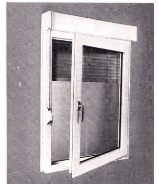
"Mini"-Rolladenelement S 732
