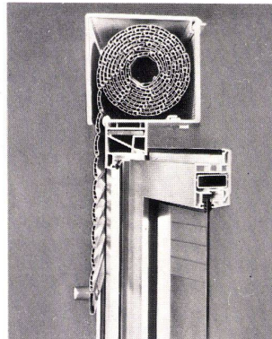
Schnitt S 732
