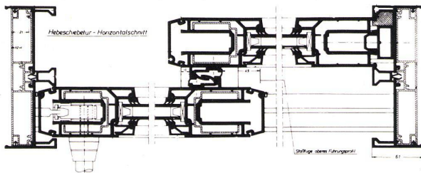
Schnitt S 732
