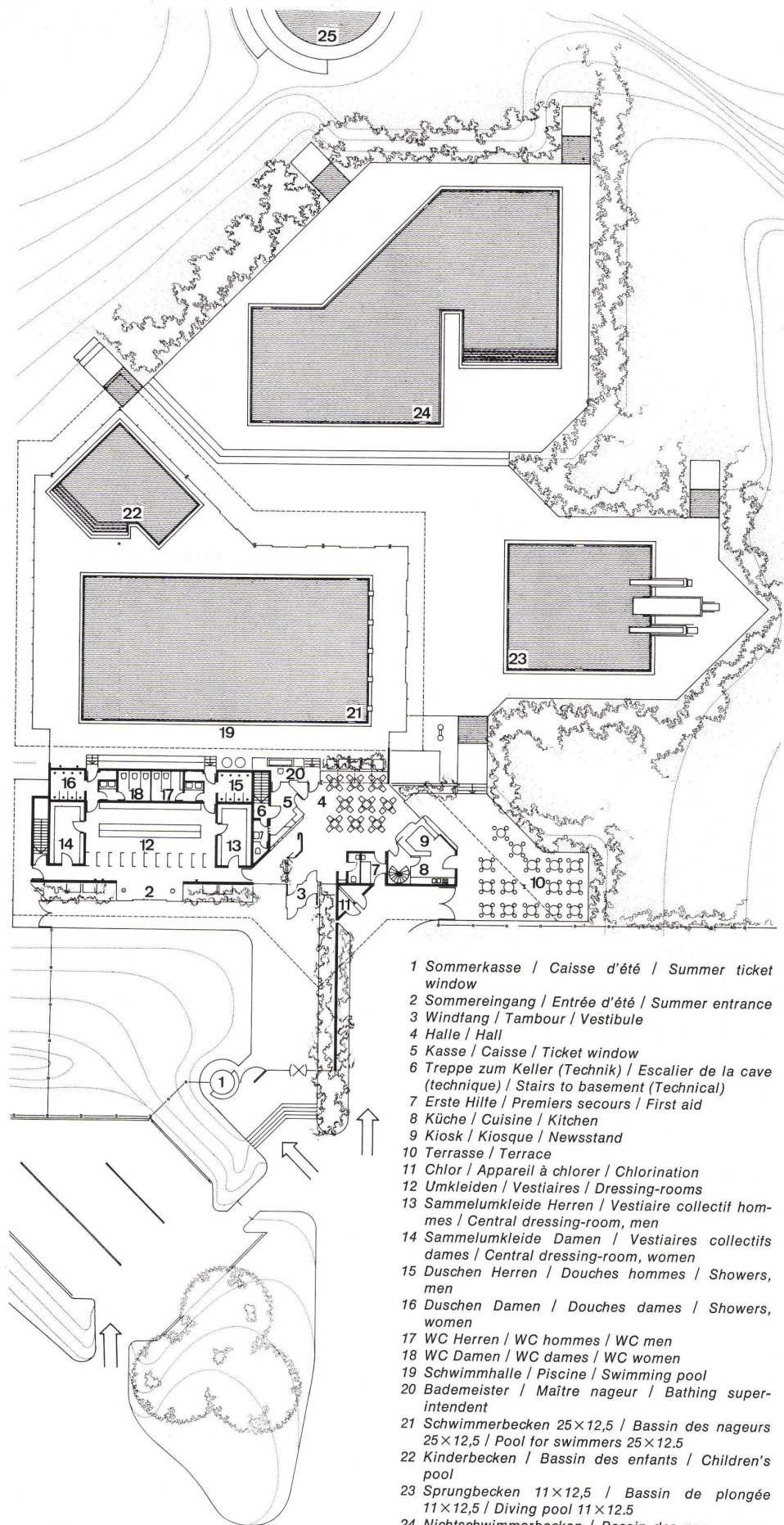
Grundriß 1:1000. Plan.
