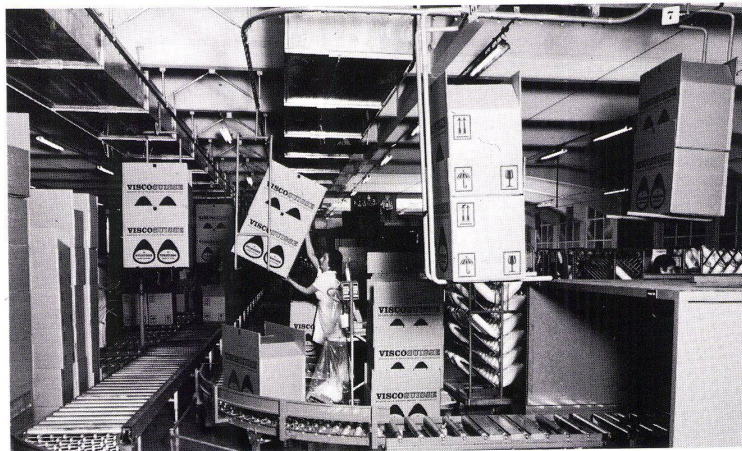
Kombinierte Förderanlage mit Rohrkreisförderer, Rollenbahnen und Förderbänder
