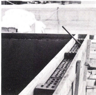
5 Einschalen Coffrer
