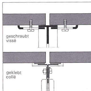
18 Stossstellen Impact du joint
