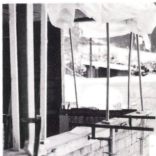
13 Verspriessen Etayer
