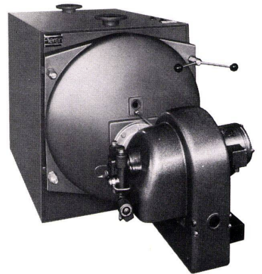
Pieren Strahlungs-Hochleistungs-Heizkessel meteor SL 18.
