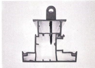
Höchste Ausreißfestigkeit ist bei GEVO dadurch gewährleistet, daß alle belasteten Schrauben durch 2 Wandungen gehen.
