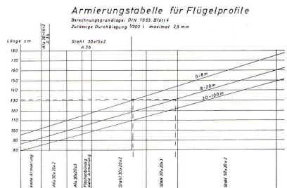
Abgestufte Armierung – das heißt: je nach Beanspruchung werden 1 oder 2 Rohre in das GEVO-Profil eingeschoben.
