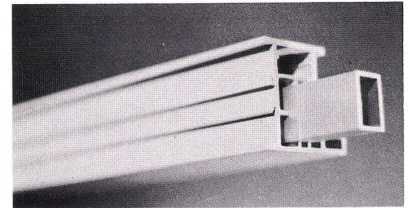
Abgestufte Armierung – das heißt: je nach Beanspruchung werden 1 oder 2 Rohre in das GEVO-Profil eingeschoben.
