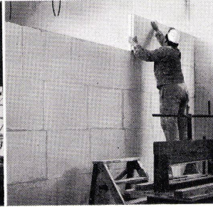
Montage Alba-Platten
