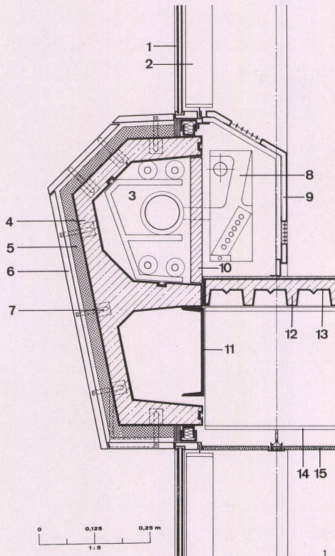
1 Brüstungsdetail. Détail d'allège. Parapet detail.
