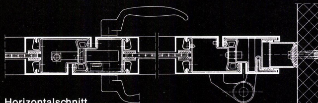
Horizontalschnitt
