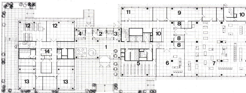
6 Großraumbüro mit quadratisch gerasterter Decke, in welche akustische, beleuchtungs- und klimatische Funktionen integriert sind. Die Möblierung stammt nicht vom Architekten.
