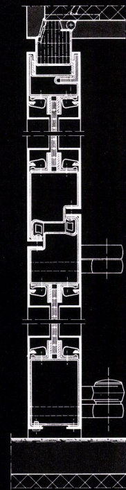
Vertikalschnitt
