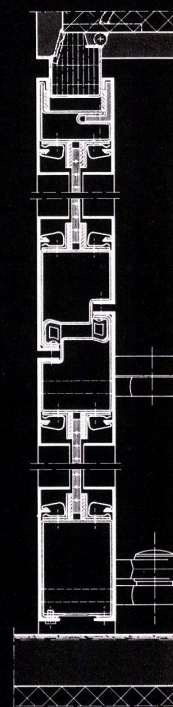
Vertikalschnitt
