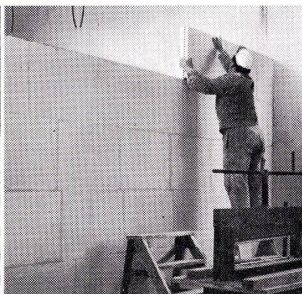
Montage Alba-Platten
