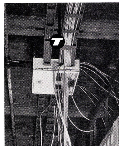
Zwischendecken-Installation
