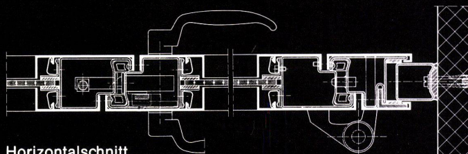
Horizontalschnitt
