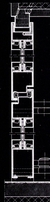
Vertikalschnitt
