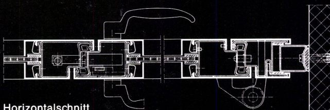
Horizontalschnitt
