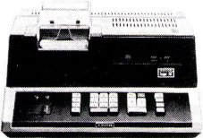
CS 661 16 Stellen. Ein Rechenspeicher. Ausgerü- stet mit neuartigem mechanischem Schnellschreiber. Konstantenvorrichtung. Druckspeicher. Kontrolllampen für freie Tastatur, für Kapazitätsüberschreitung und Belegung des Rechenspeichers. 38 x 18 x 43 cm. 12 kg. Fr. 4390,-
