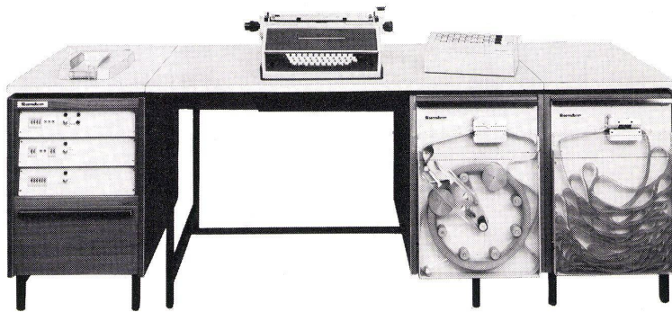
Addo-Forster 2500 – ein Korrespondenz- und Organisations-Automat für integrierte Arbeitsabläufe ab Lochstreifen, Lochstreifen-Karten und Lochkarten. Eine logische Konzeption in der Datentechnik.
