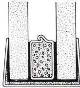
POLYGLASS Isolierglas mit elastischer Dichtung in einem starren Rahmen. Vielseitige Kombinationsmöglichkeiten. Produkt Glaceries de Saint Roch (Belgien)
