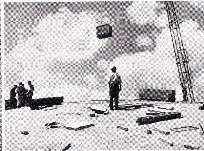
Buckelschalung mit Perfecta-Platten
