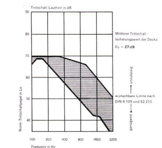
Trittschalldämmung eines Hartbelages samt Isolation und schwimmendem Boden
