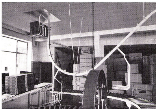
Kreisförderanlage für Stückgüter mit Abgabe-Rollenbahn
