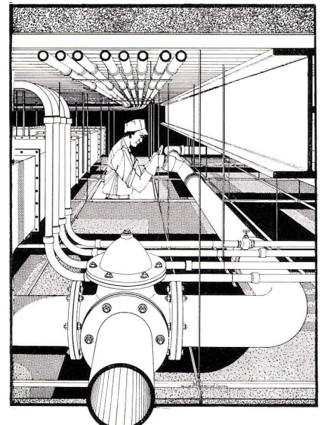
Jede Platte kann einzeln ausgewechselt werden. Der Deckenhohlraum ist an jeder Stelle zugänglich.
