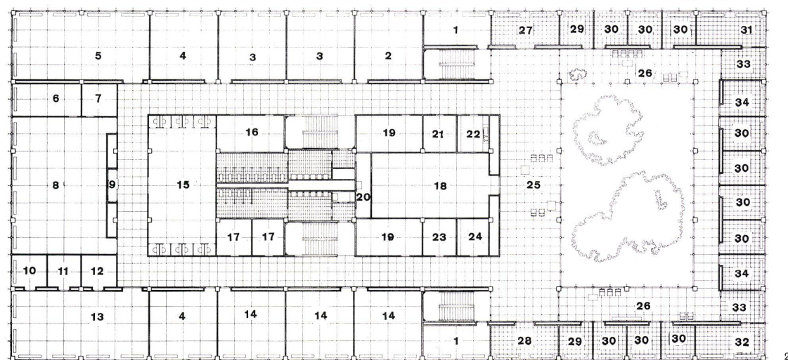
1 Grundriß Erdgeschoß 1:500. Plan rez-de-chaussée.
